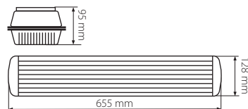
● DICT-218/PC/PS
