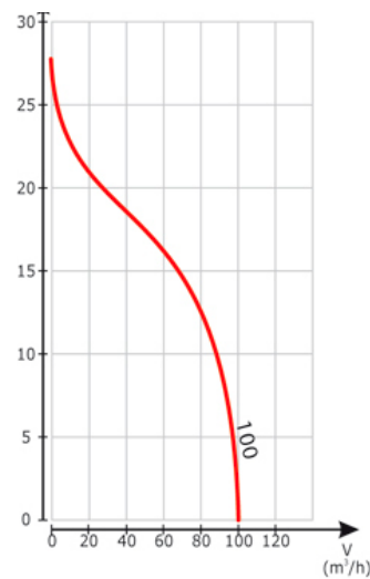
Charakteristika ventilátoru Charakteristika ventilátora
